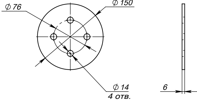
Поз.4 (Диск)
