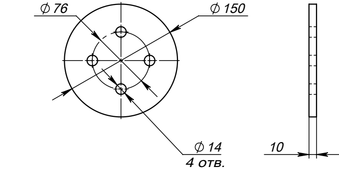
Поз.4 (Диск)
