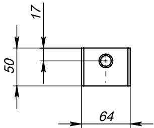
Поз.2 (Пластина)
