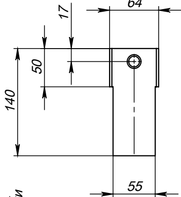
Поз.6 (Пластина)
